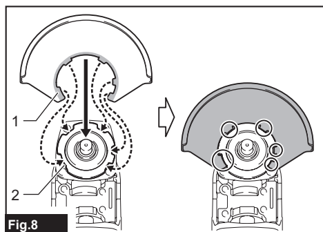
Fig. 8 ► 1. Protrusion 2. Notch
