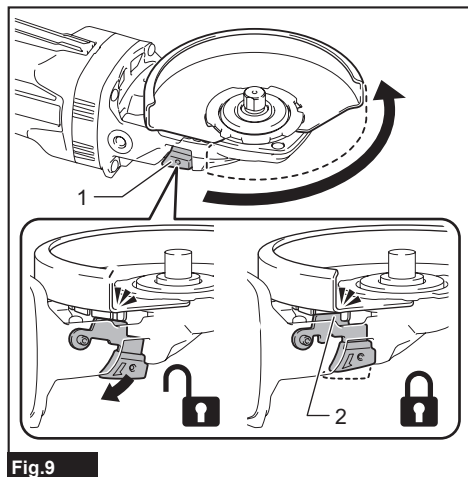
Fig. 9 ► 1. Lock lever 2. Groove
