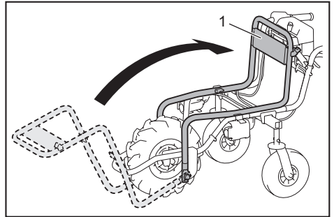
► 1. Carrier frame
